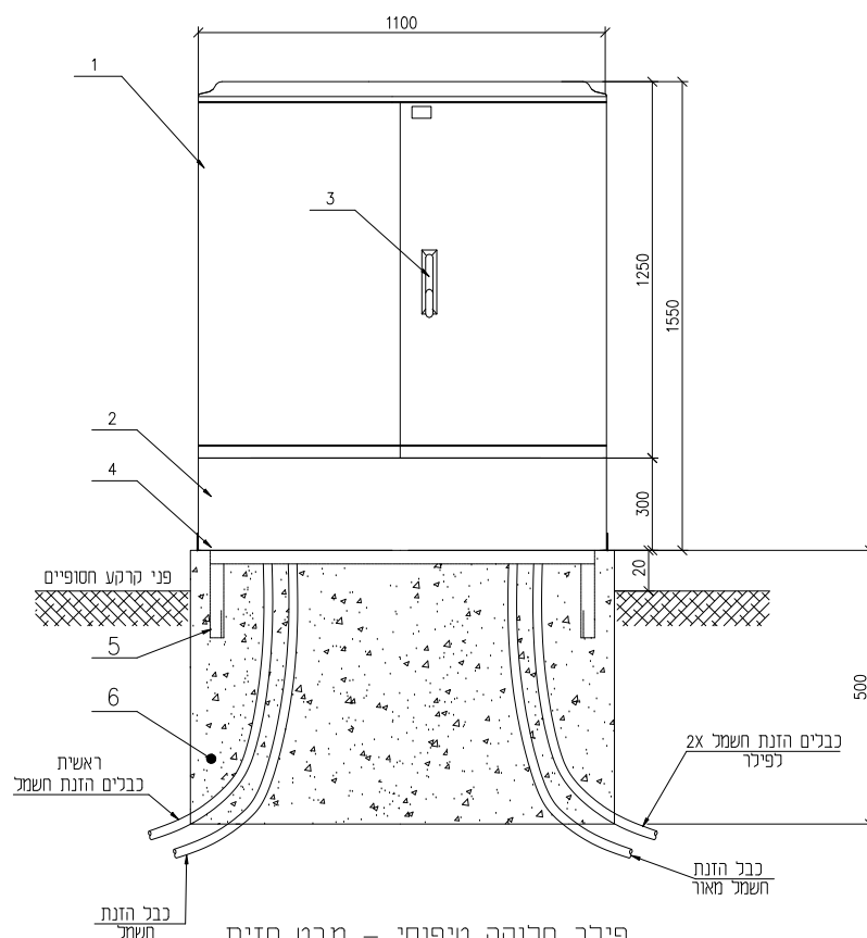
פילר חלוקה טיפוסי – מבט חזית ללא ק.נ.מ.
