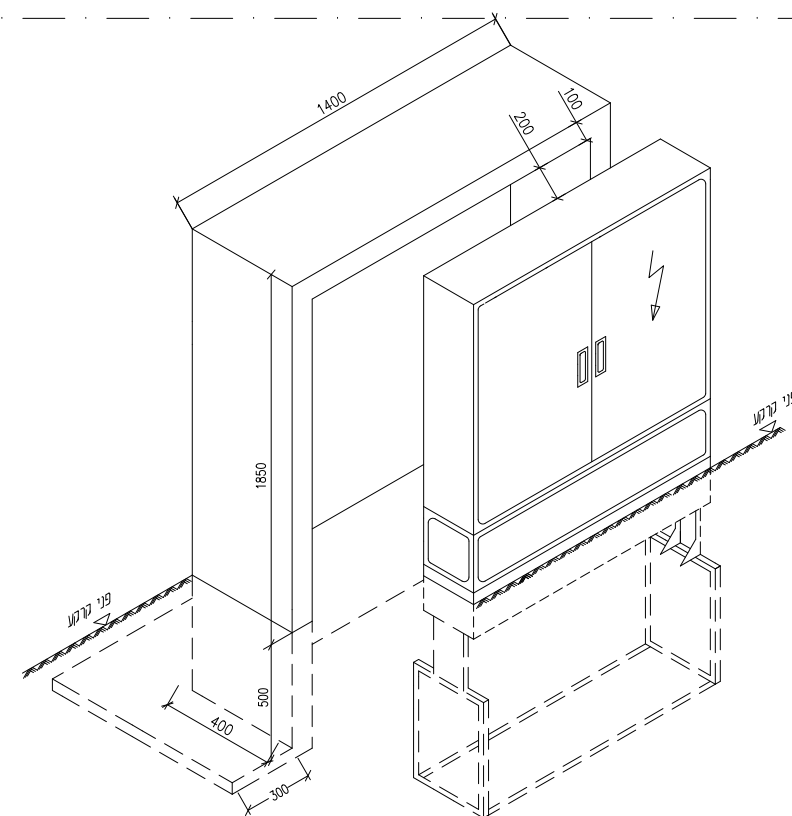
פרט גומחה לפילר ללא ק.נ.מ.
