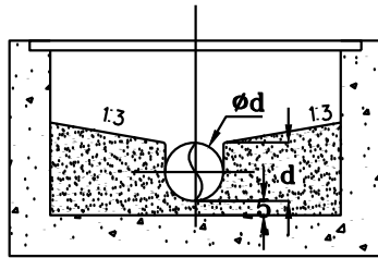
חתך ג-ג
