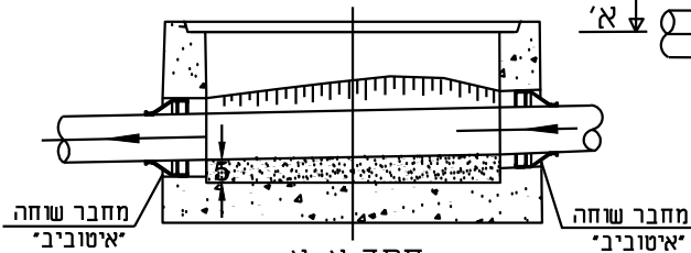
חתך א-א
