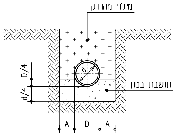
תושבת בטון
