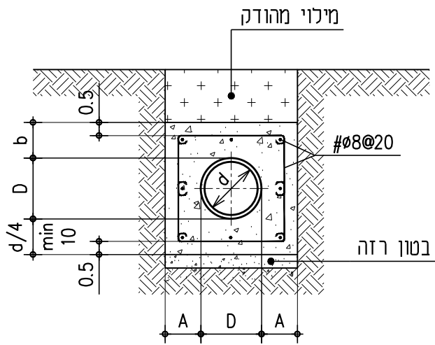
עטיפת בטון מזוין
