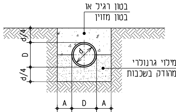
כיסוי בטון קשתי
