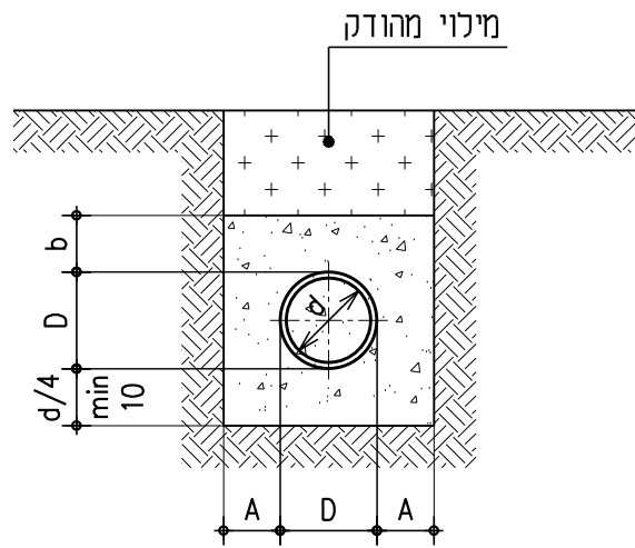
עטיפת בטון
