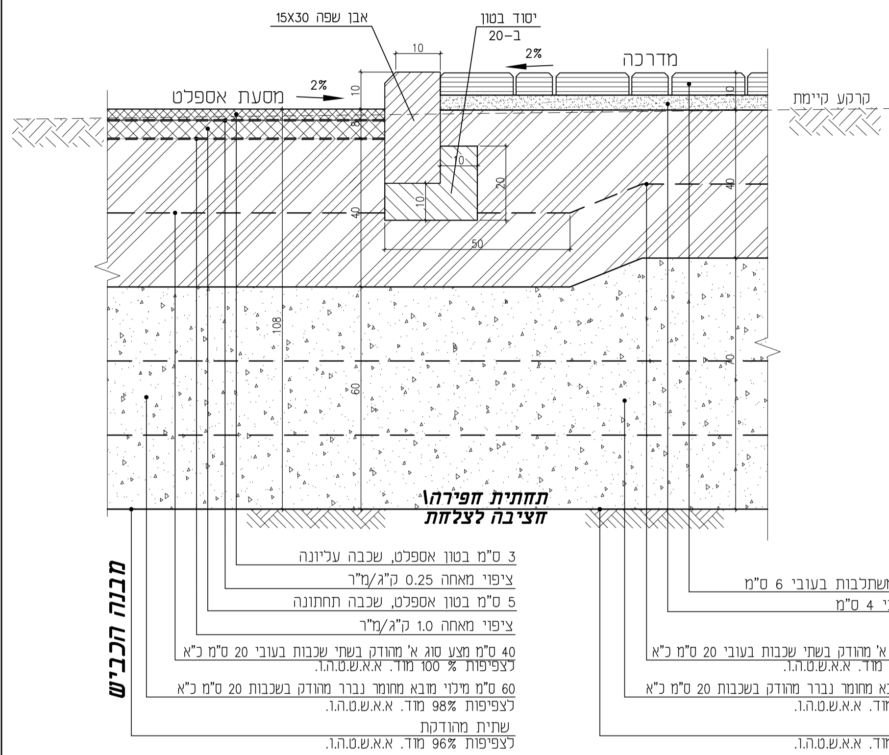
פרט מבנה כביש, אבן שפה ומדרכת אבן משולבת קנ"מ 1:10
