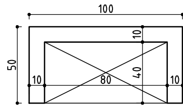
A גומחה לחוני חשמל ארון רשת גודל 0 מידות פנים 80x40 ס"מ גובה פנים 150 ס"מ מעל פני הקרקע
